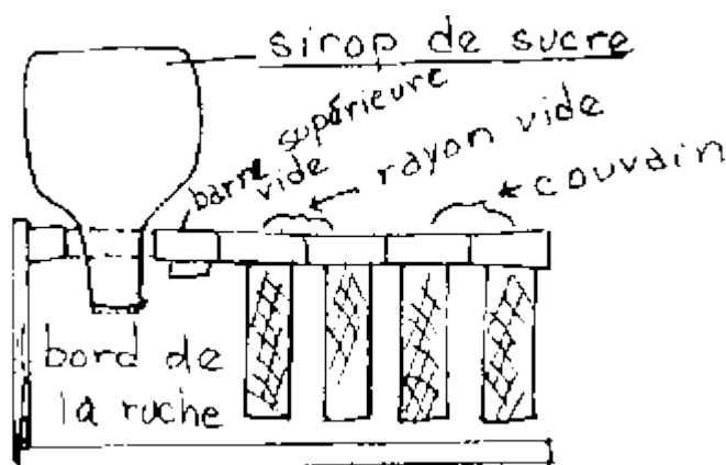
Appareil à alimenter de la KTBH (vue latérale en longueur)
