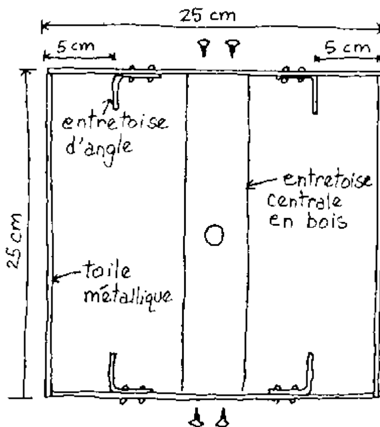
Vue d'en haut de la cage
