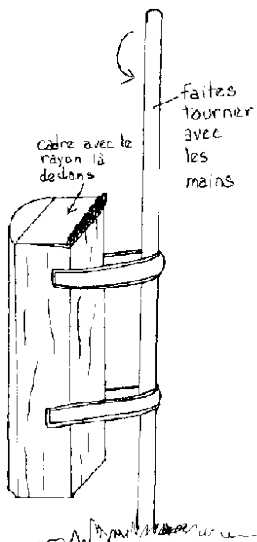
Extracteur de miel manuel
