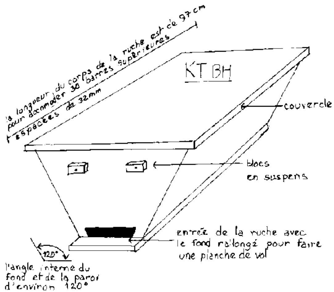
Ruche à barres supérieures du Kenya (= Kenya Top Bar Hive = KTBH) Dimensions en cm, basées sur des planches de 1,9 cm d'épaisseur
