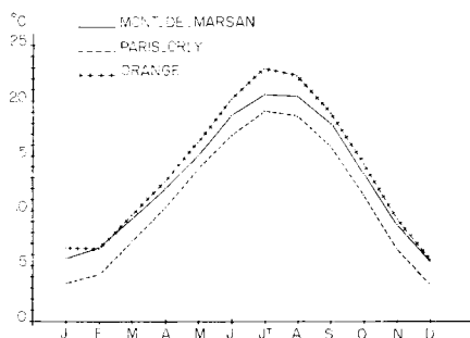
FIG. 2. — Températures moyennes à Mont-de-Marsan, Paris-Orly et Orange. Moyennes trentennaires établies par la Météorologie nationale.
